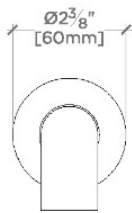
FRONT VIEW SCALE: 3"=1'-0"
