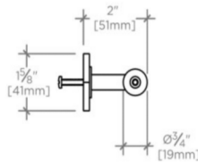
SIDE VIEW SCALE: 3"=1'-0"
