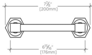
FRONT VIEW SCALE: 3"=1'-0"
