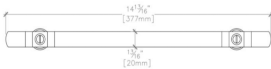
FRONT VIEW SCALE: 3"=1'-0"
