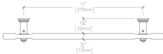
TOP VIEW SCALE: 3"=1'-0"
