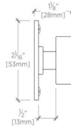
SIDE VIEW SCALE: 6"=1'-0"
